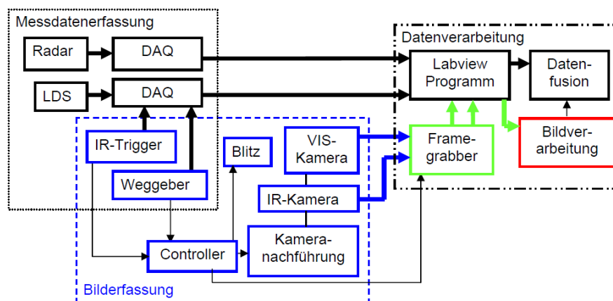
Abb. 17: Signalverlaufdiagramm für die Sensorik am Ausleger aus dem Artikel: Untersuchungen zur Wilderkennung beim Mähen
