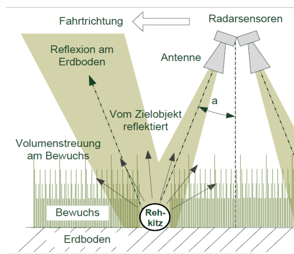
Abb. 18: Doppelradar-Prinzip Aus dem Artikel: Untersuchungen zur Wilderkennung beim Mähen
