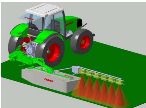
Abb. 15: Prinzipbild Sensorträger (Ausleger)
